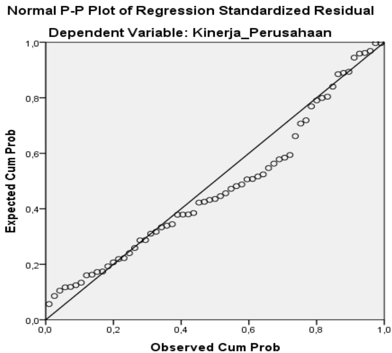
Gambar 5.1 Grafik P Plot sebelum Normal
