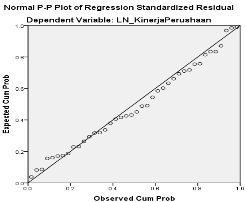
Gambar 5.2 Grafik P-Plot Setelah Normal
