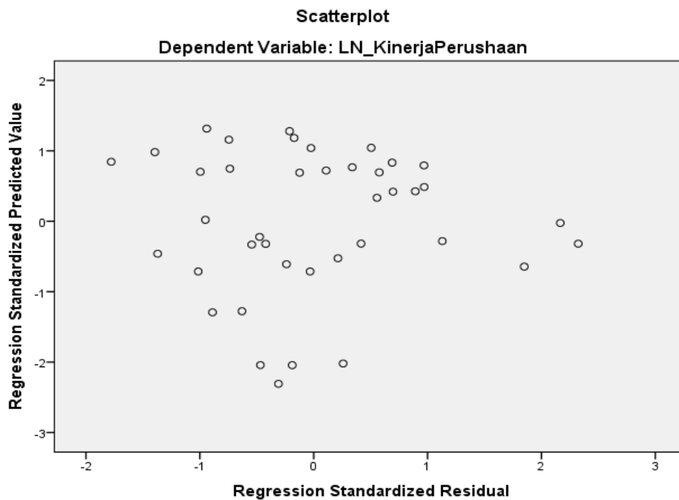
Gambar 5.3 Grafik Scatterplot
